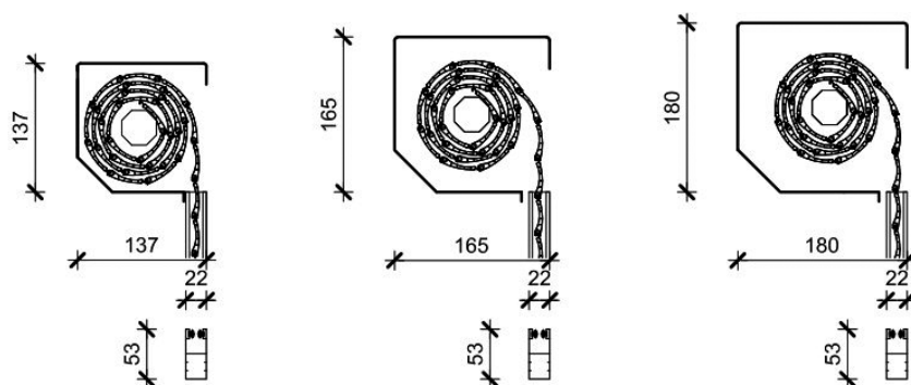
Külső redőnytok méretek
